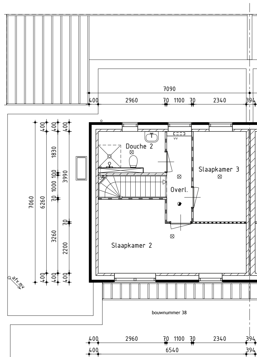
1ste Verdieping
