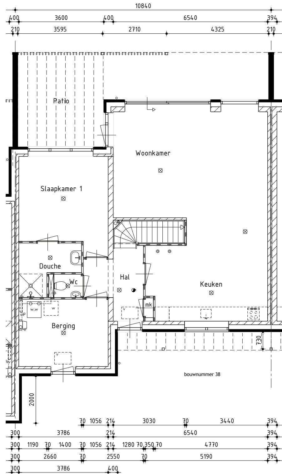
Begane grond
